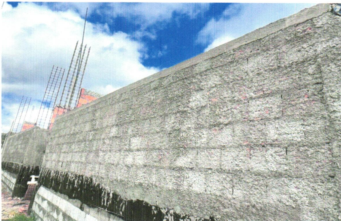
FOTO 24 – Verga e contraverga pré-moldada fck= 20MPa, seção 10x10cm
