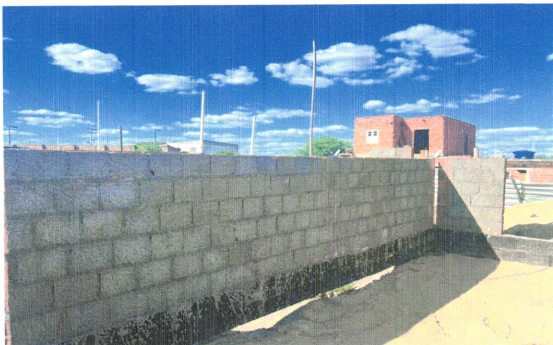
FOTO 42 – Chapisco de aderência em paredes internas, externas, vigas, platibanda e calhas
